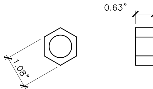
NUT X2
