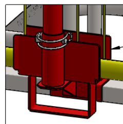
GUIDE POST 08051541-1
