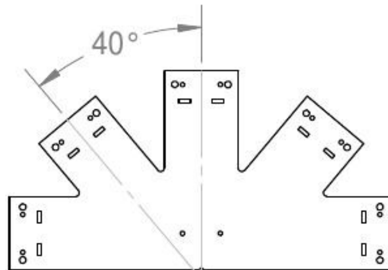
56620 10:12 Truss Base Fan
