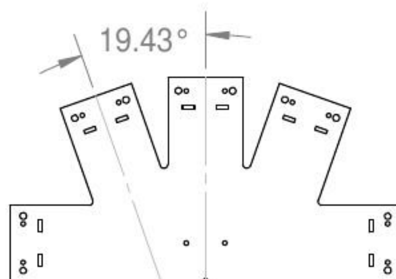
56642 4:12 Truss Base Fan
