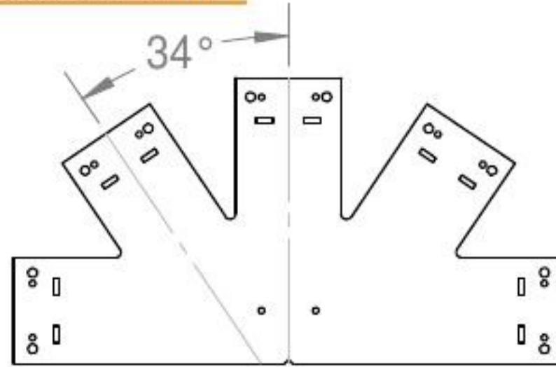
56619 8:12 Truss Base Fan
