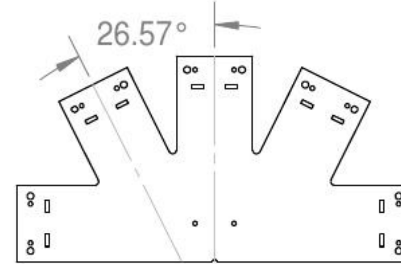
56643 6:12 Truss Base Fan
