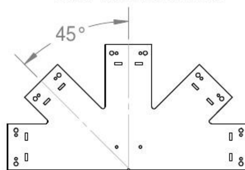
56644 12:12 Truss Base Fan
