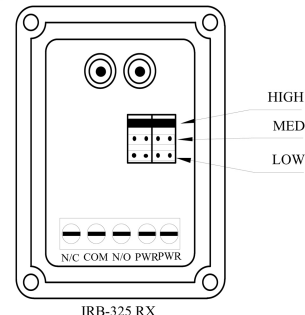
IRB-325 RX
