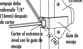
Parte trasera del poste de la cerca
